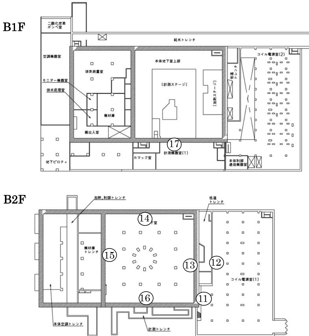
図 3-2-1 (2) 大型ヘリカル実験棟での測定位置
