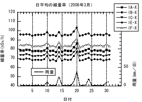
図 3-3-5 (3) 日平均の線量率データ 3 (12月-3月)
