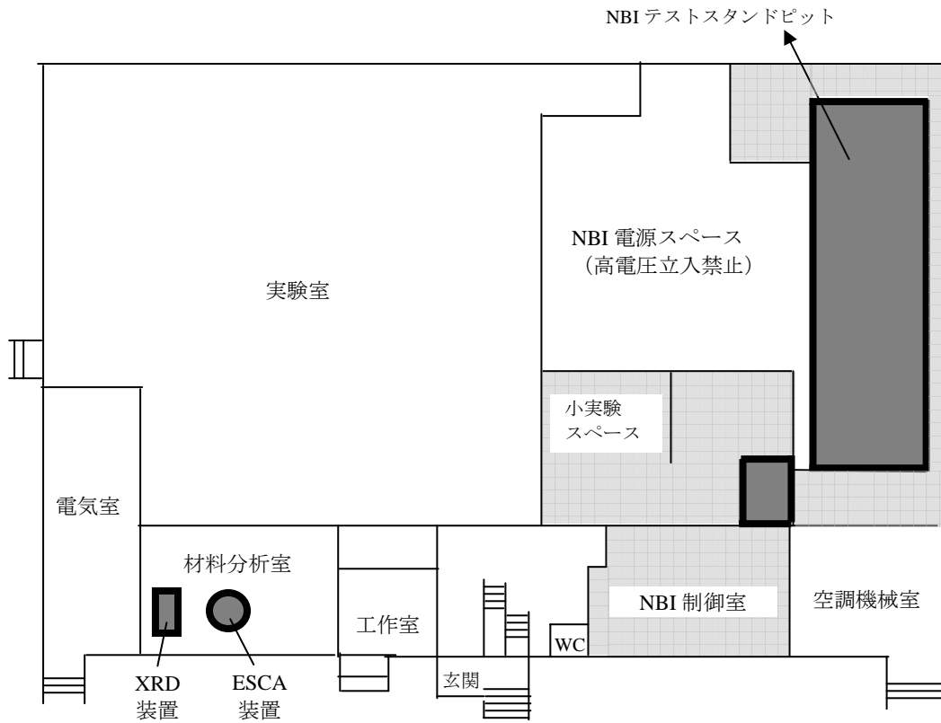
図 1 - 3 - 2 総合工学実験棟の装置管理区域と装置監視区域 (2007 年度末現在)
