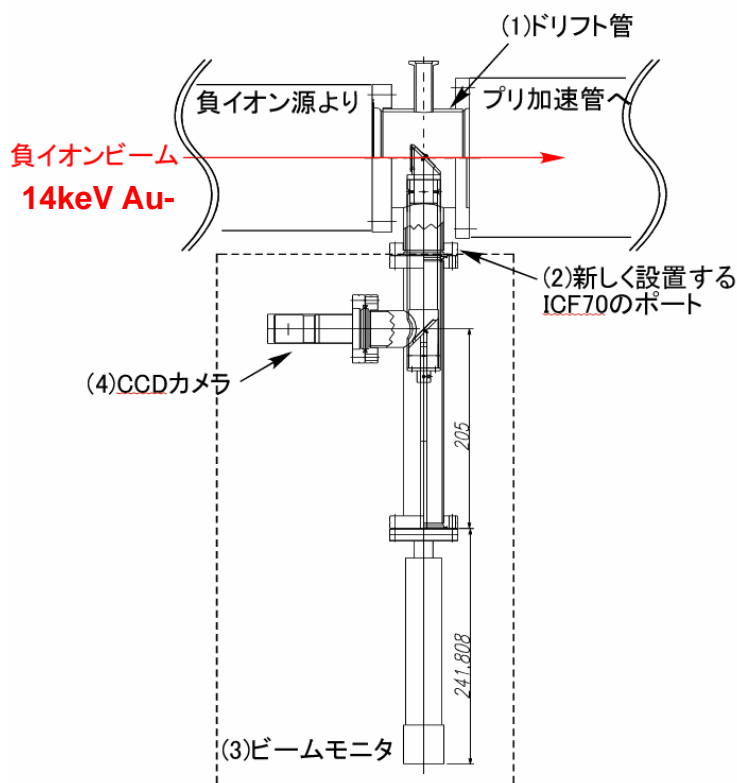
図 4-1 ビームモニターの追設内容
