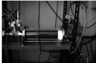
Fig.3. Ar discharge
