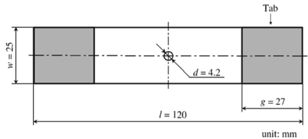
Fig. 1. Open hole specimen.
